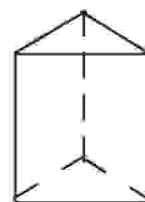
ପ୍ରିଜମ୍
