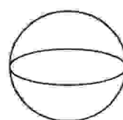
ଗୋଲକ
